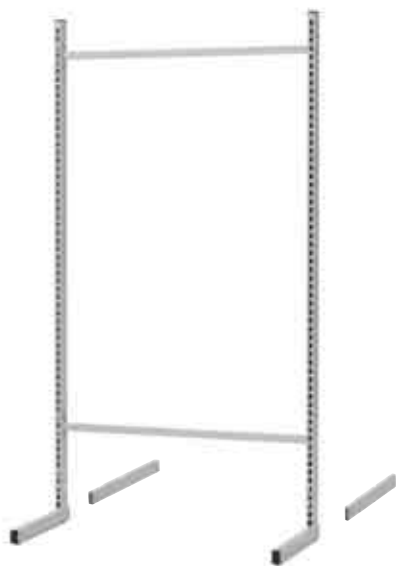
Стойка напольная 1500 x 900 x 410 мм Артикул 9011.830.501
